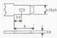
Optional Terminal F2 (Fasten Tab No.250A)
